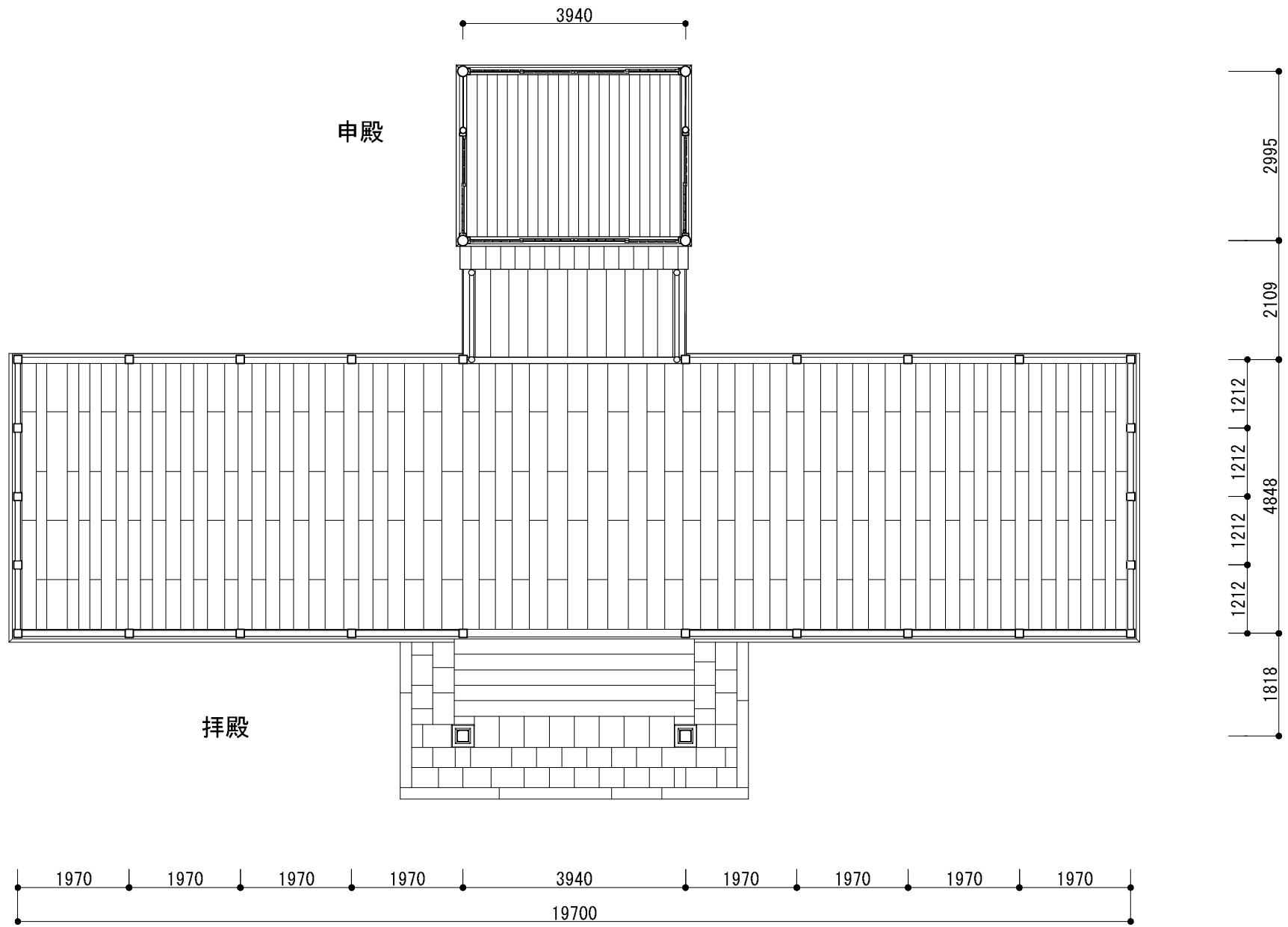
捍殿·申殿 平面图 1:100
