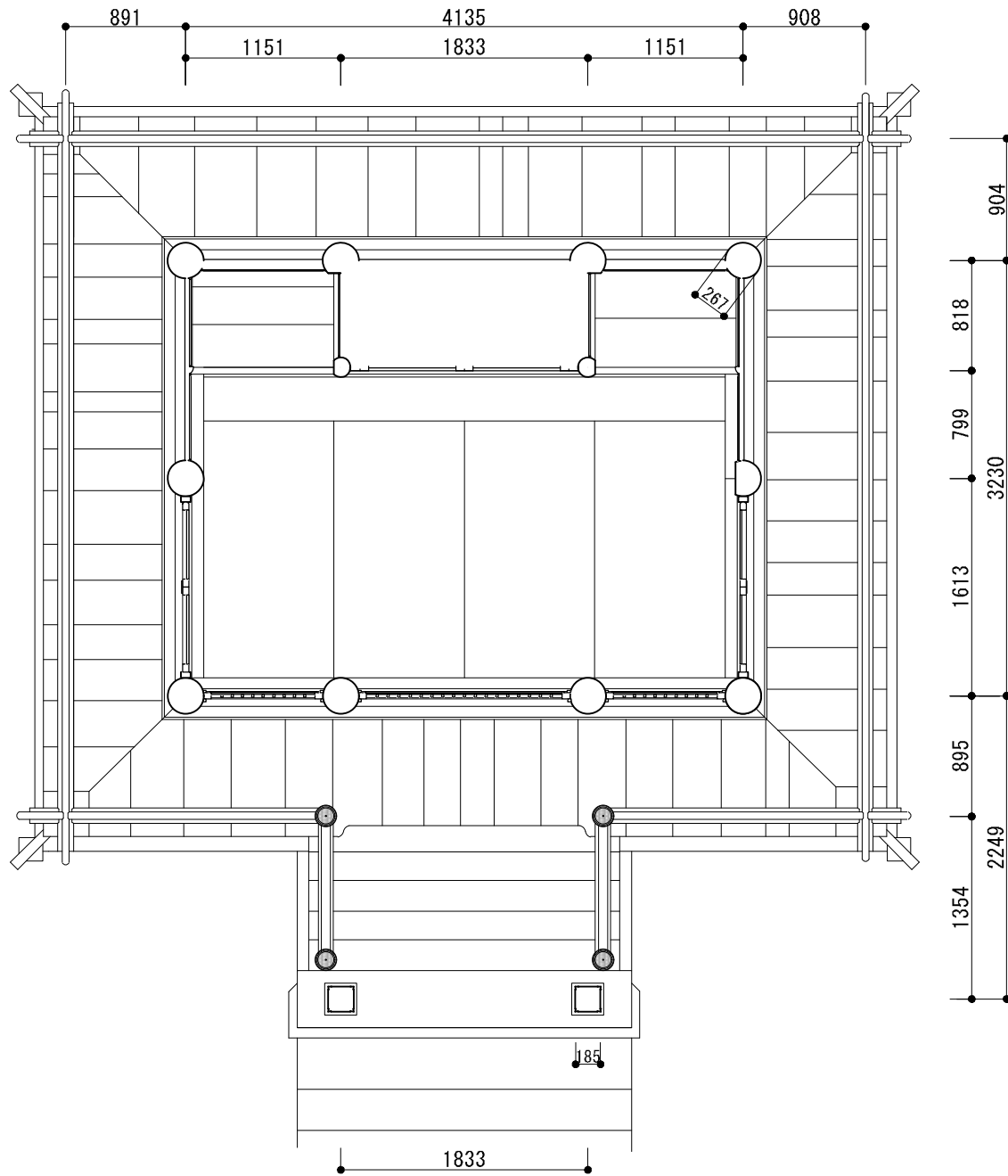
本殿（神殿） 平面図 1:50
